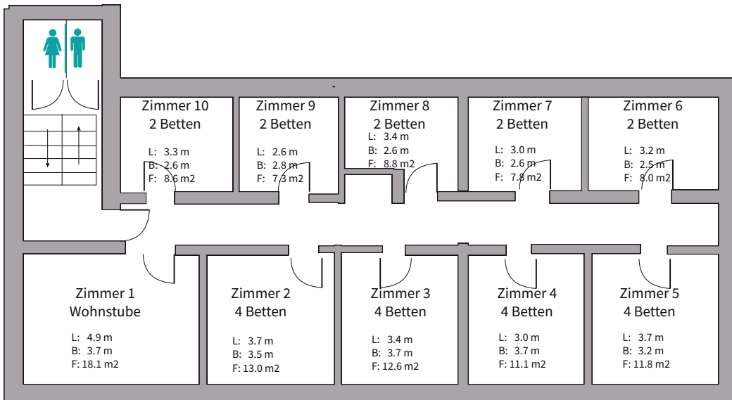
1. Obergeschoss
