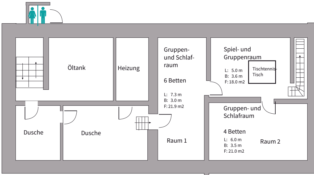
Kellergeschoss
